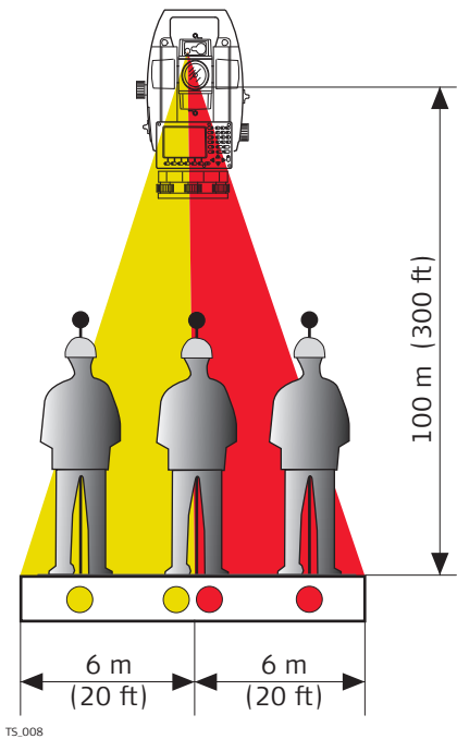
TS_008
